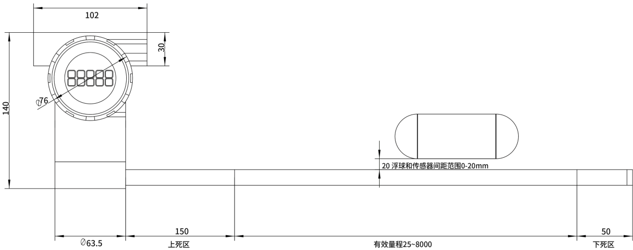
捆绑式 外形尺寸
